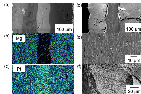
金属蒸気の選択反応による貴金属回収 Metal vapor treatment for precious metal recovery
