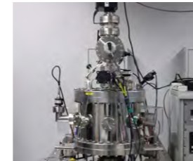
高温質量分析装置を利用した 材料製造プロセスのための反応解析 Reaction analysis of material production processes by high-temperature mass spectrometry
